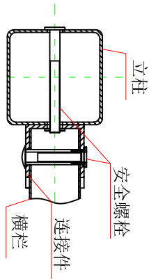
栅栏与立柱连接方式
